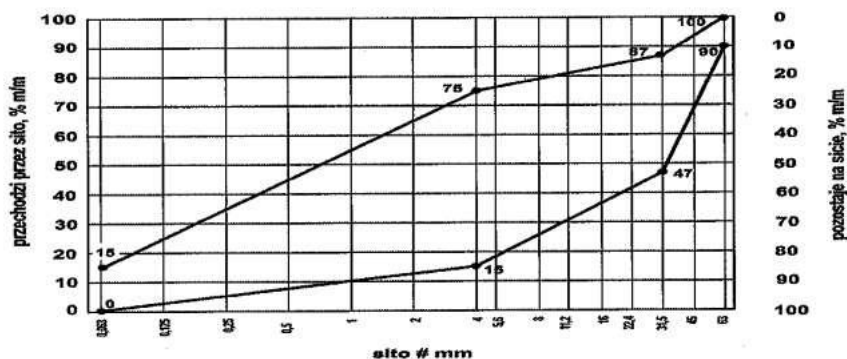
Rys. 8. Mieszanka kruszyw 0/63 do górnej warstwy podłoża ulepszonego
