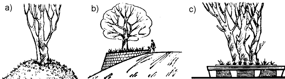
a) pozostawiony ścięty stozek z gruntu, ochraniający korzenie drzewa b) ścianka podporowa z kamienia wokół drzewa pozostawionego na skarpie c) ścianka oporowa dostosowana do odpoczynku podróżnych przez wykonanie ławki na jej górnej powierzchni
