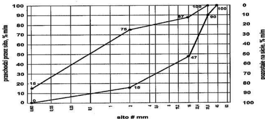
Rys. 6. Mieszanka kruszyw 0/31, 5 do górnej warstwy podłoża ulepszonego
